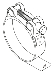
Конструкция силовых хомутов ROBUST SR/W2
