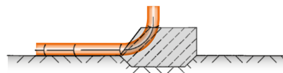
Рис. 9 Фиксация трубопроводов
