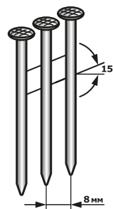
Гвозди в обойме на сварочной проволоке
