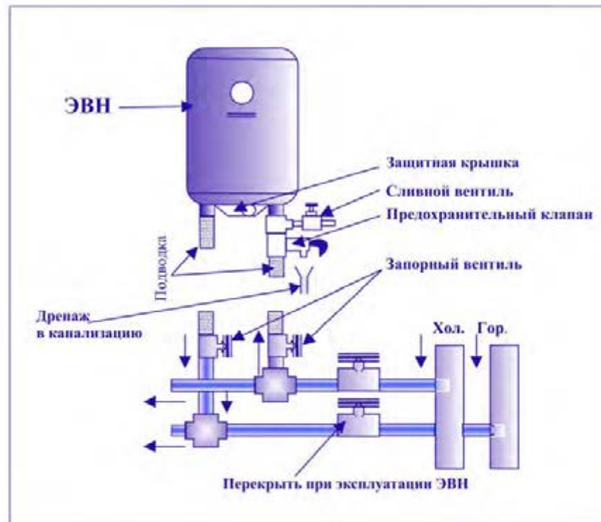
Рис. 1. Схема подключения ЭВН к водопроводу
