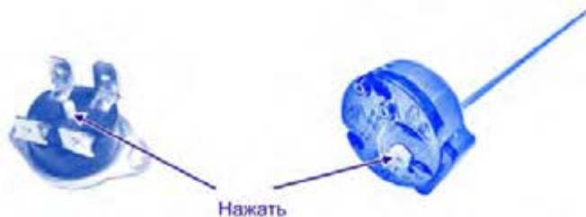
Рис.2. Расположение штока на термовыключателе термостата
