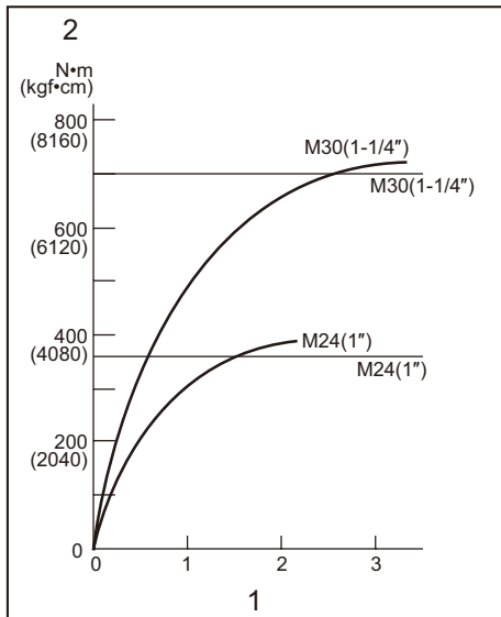
1. Åtdragningsmoment 2. Åtdragningsmoment
