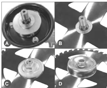
Рис. 5 Установка ножа
