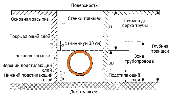
Рис. 3 Устройство траншеи
