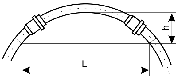
Рис. 2 Изогнутый трубопровод
