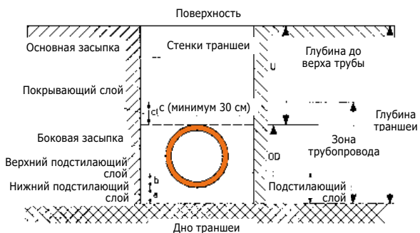
Рис. 3 Устройство траншеи
