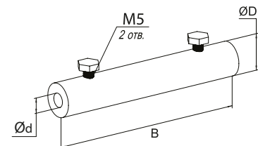
Зажим продольный
