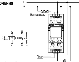
Рис. 3 Схема подключения
