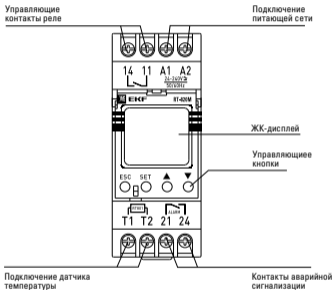
Рис. 1 Лицевая панель
