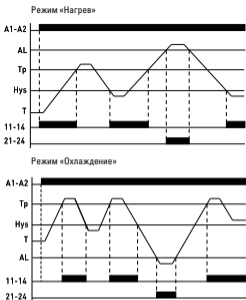
Рис. 2 Диаграммы работы реле
