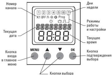
Рис. 1 Лицевая панель
