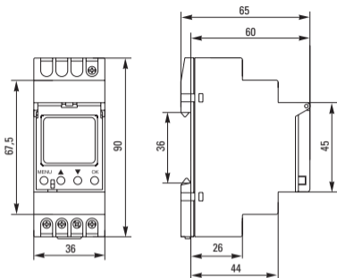
Рис. 3 Габаритные и установочные размеры
