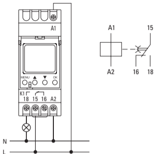
Рис. 2 Схема подключения
