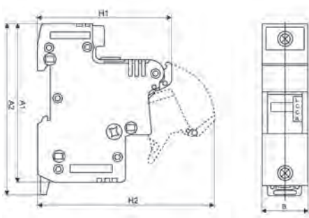
Габаритные размеры предохранитель-разъединителя
