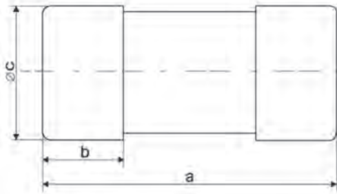
Габаритные размеры плавких вставок ПВЦ
