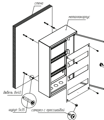
Рис.1. Схема монтажа
