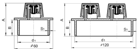
Рис 2.Аэраторы d 50 и 110 мм.
