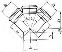
Рис 4. Крестовина одноплоскостная
