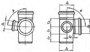
Рис 5.1. Крестовина двухплоскостная
