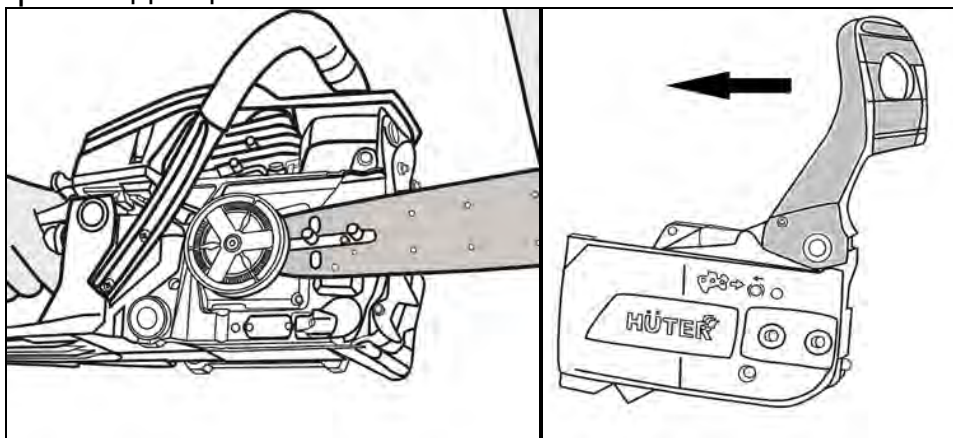
Рис. 5. Установка шины
