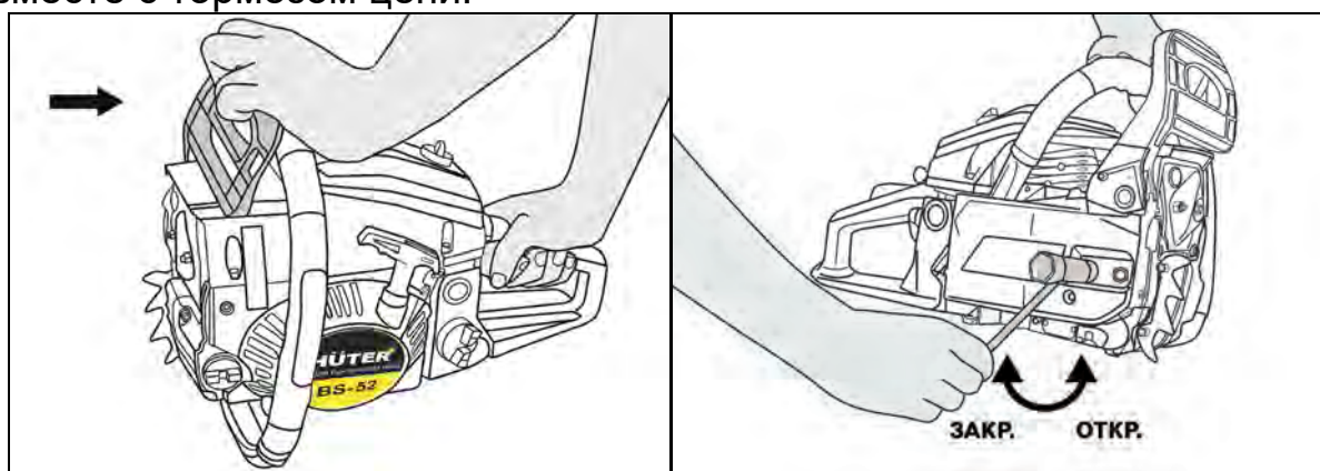
Рис.1 Ослабление гайки прижимной крышки шины
