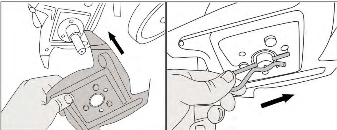
Рис. 5. Установка фрез
