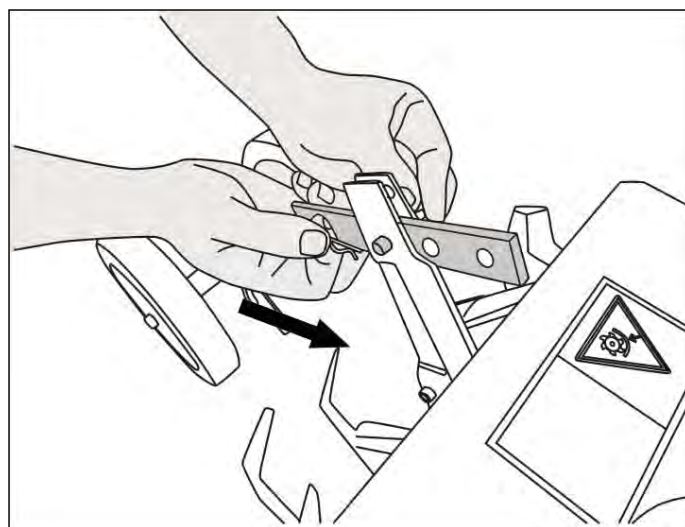
Рис. 6. Установка сошника
