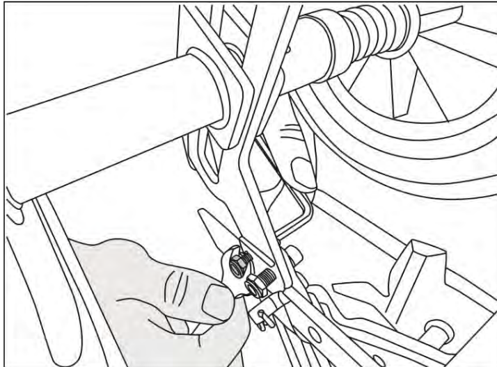
Рис. 7. Фиксация кронштейна с колесами
