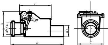
Рисунок 14. Обратные клапана
