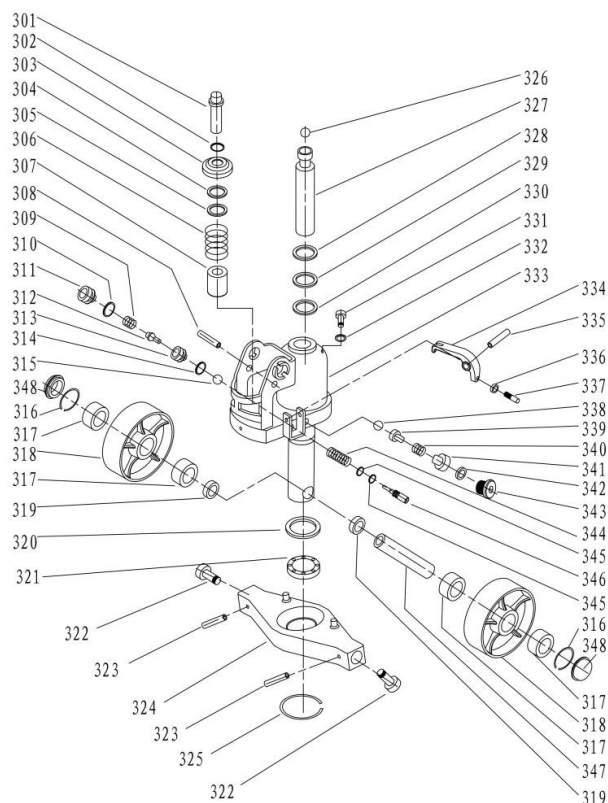
Схема 3. Взрыв-схема гидроузла тележки JC.
