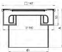
Рисунок 12. Трапы с вертикальным выпуском
