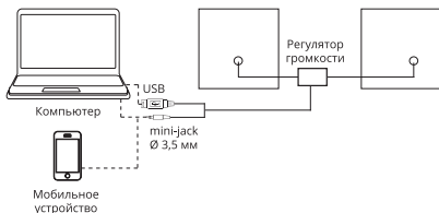
Рис. 1. Схема подключения
