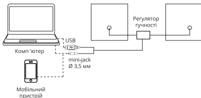
Мал. 1. Схема підключення
