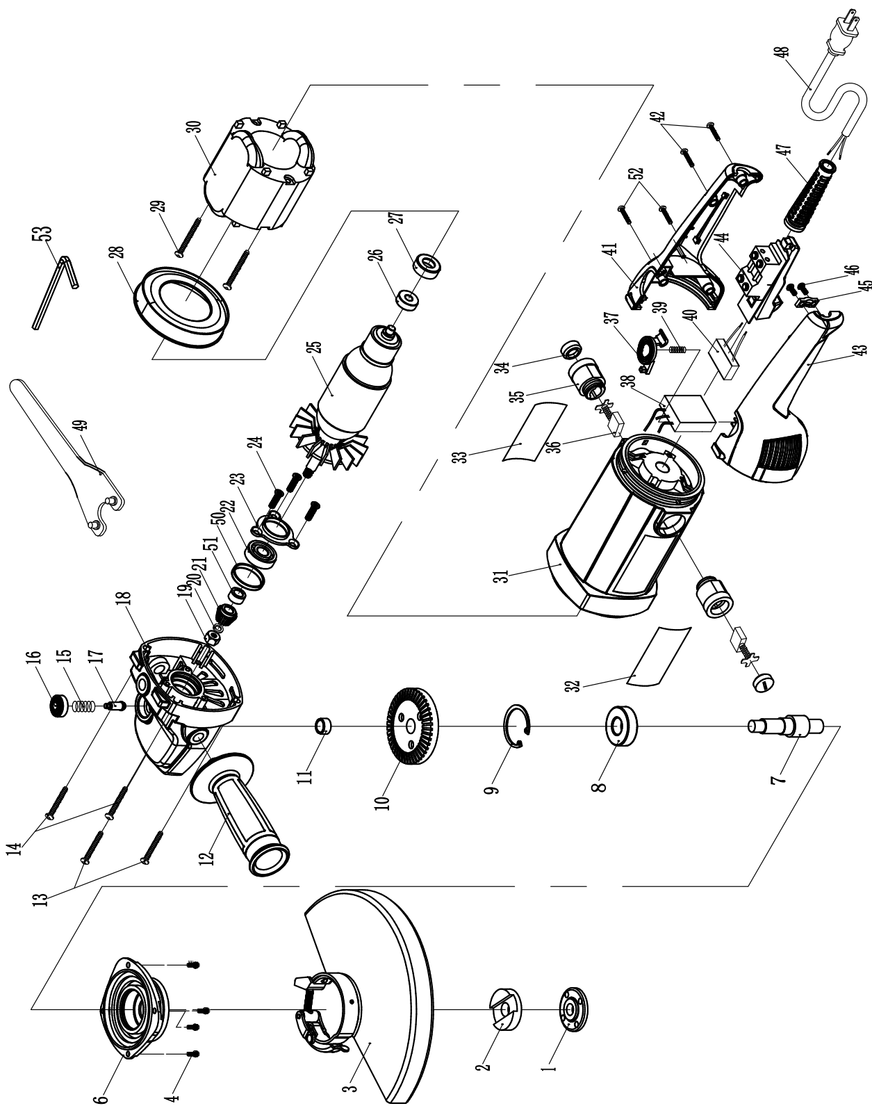
WT8508角向磨光机爆炸图 (FELISATTI 专用)
