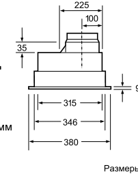
Размеры в мм
